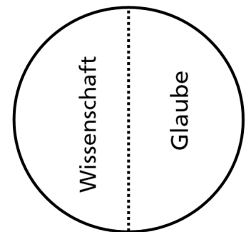
Das Dialogmodell
