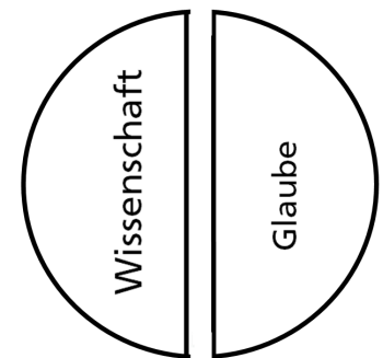
Das Trennungsmodell
